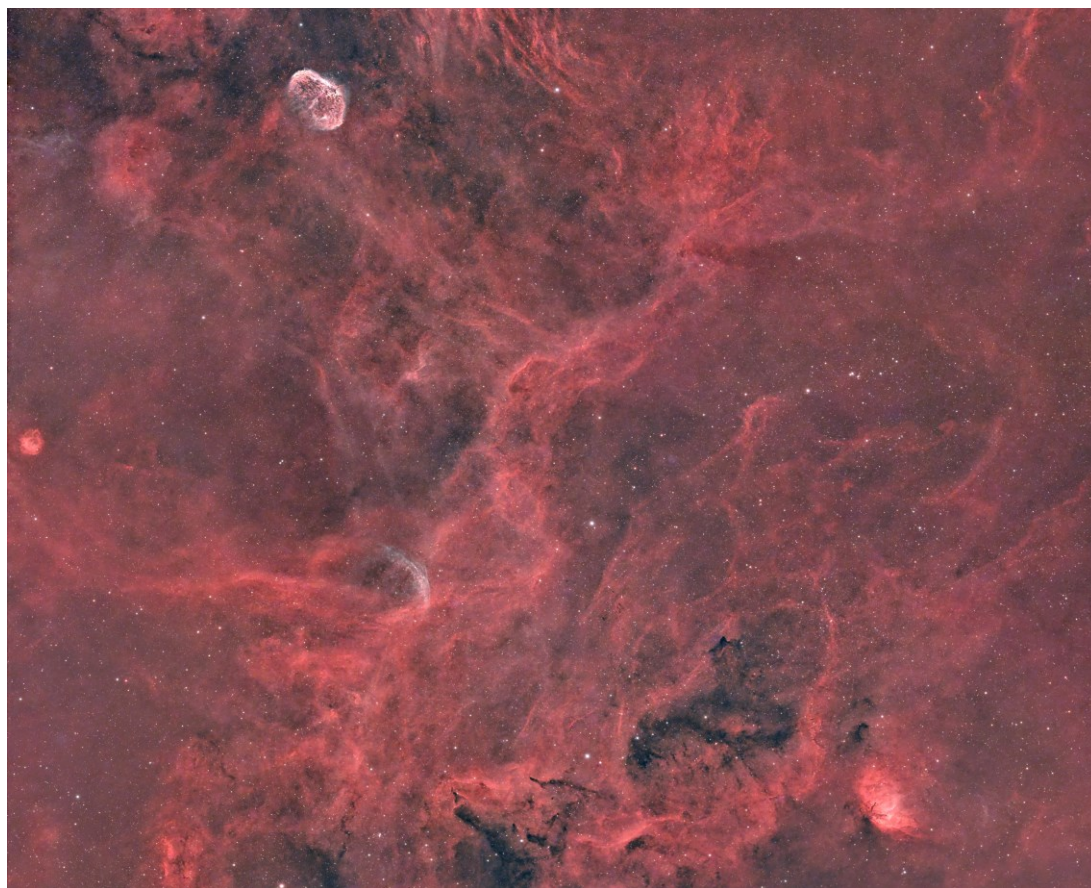
Plaga nebule nel Cigno (con nebulose "Crescent" e "Tulipano") - Carpinello FC Foto di Loris Ferrini
