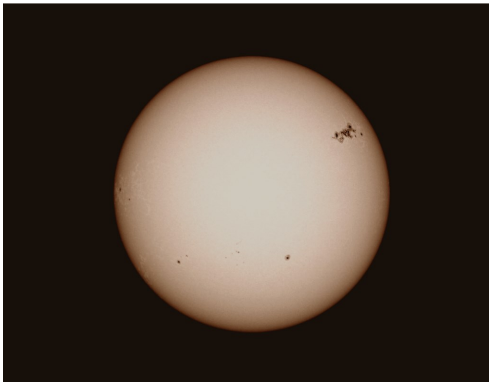
Sole con gruppo di macchie che hanno generato l'aurora del 10 maggio 2024 - Sogliano al Rubicone FC Foto di Roberto Turci
