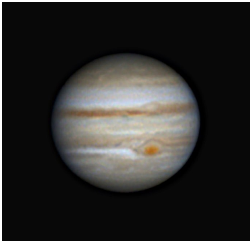
Giove con macchia rossa, 31 ottobre 2022 - Forlì
